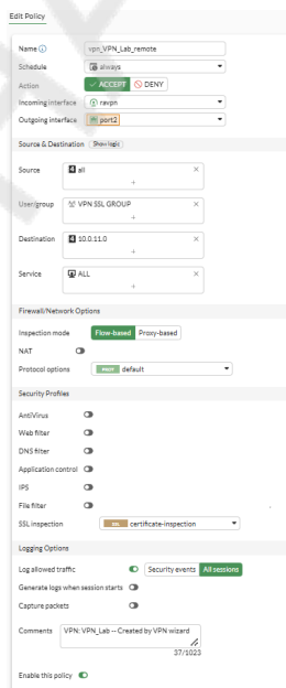
Fig. 6 - 4.6 Política vpn_VPN_Lab_remote: ravpn → port2, sin NAT, log de todas las sesiones.
